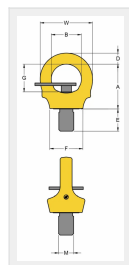
Plano de dimensiones
