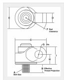
Plano de dimensiones
